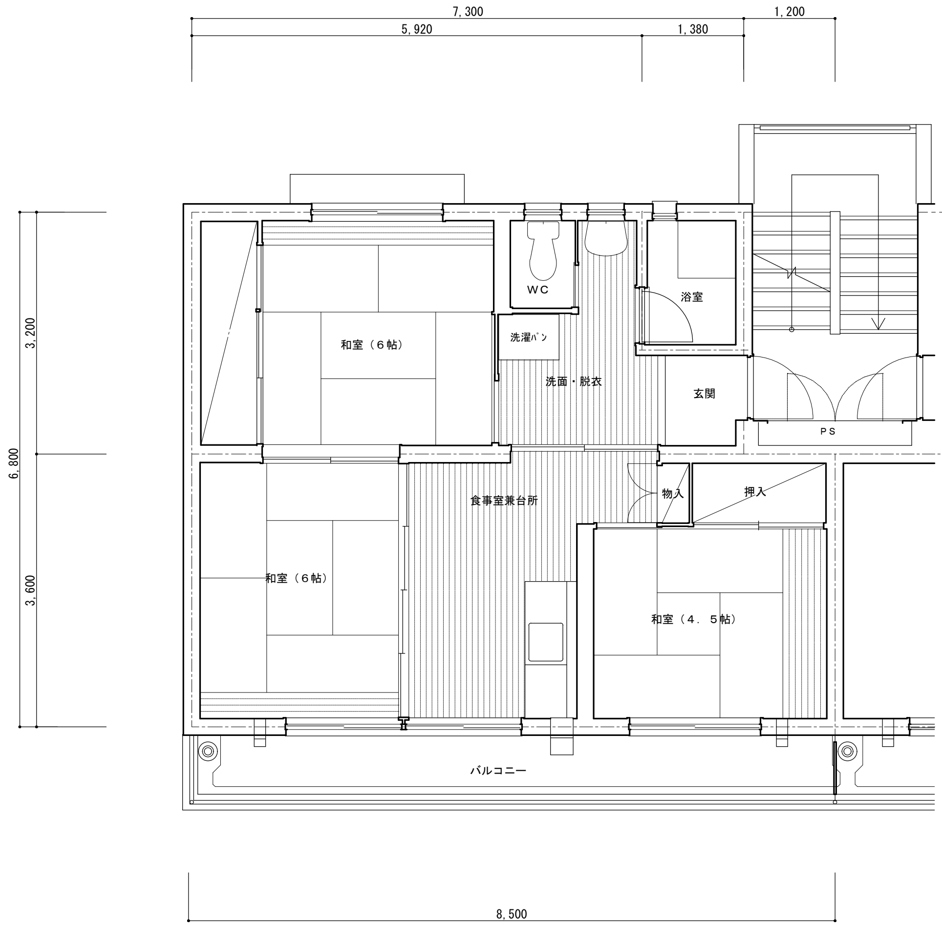
平面図 住居専用床面積 53.96㎡
