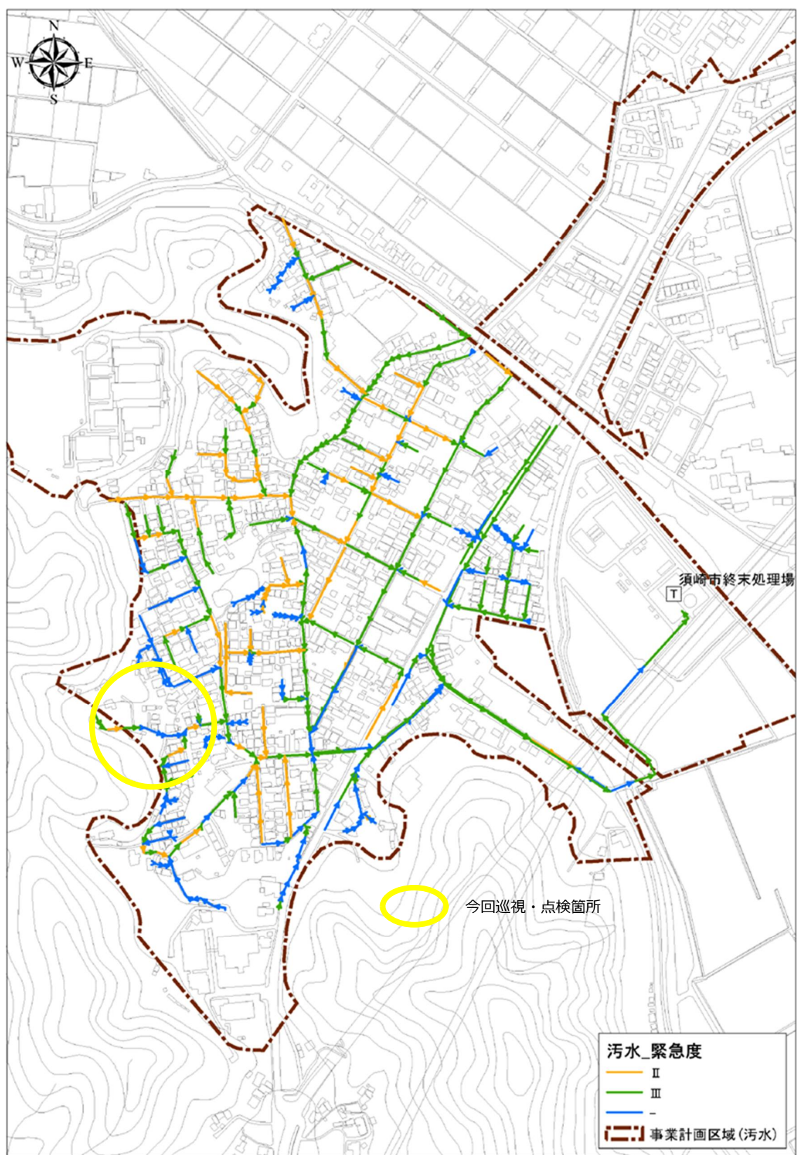
図 5-6 汚水管路 巡視・点検位置図（全体図）
