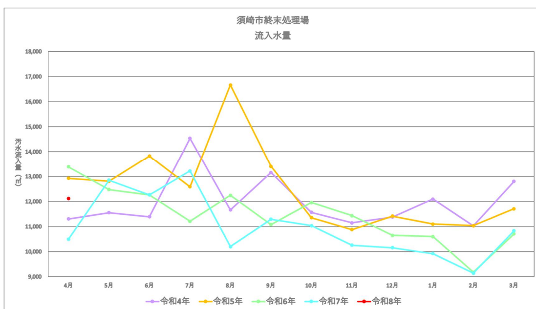
図 5-14 須崎市終末処理場の月別流入水量の推移
