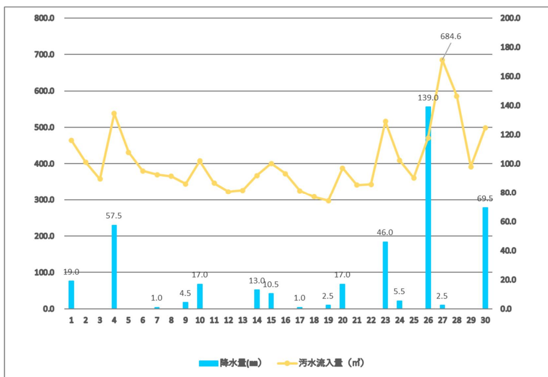
図 5-13 須崎市終末処理場の流入水量（令和 8 年 4 月）
