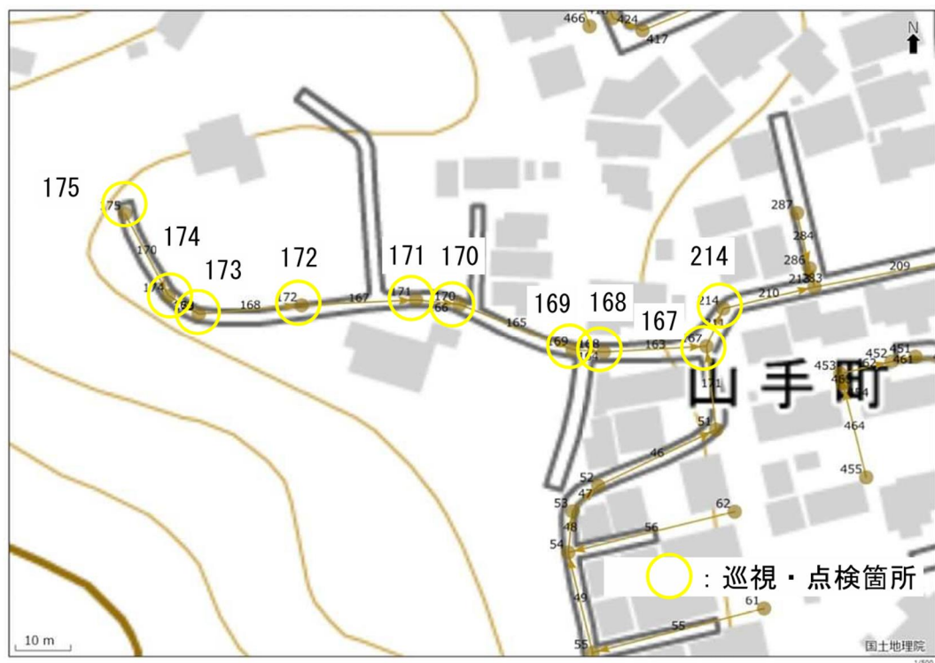
図 5-7 汚水管路 巡視・点検位置図（詳細図）
