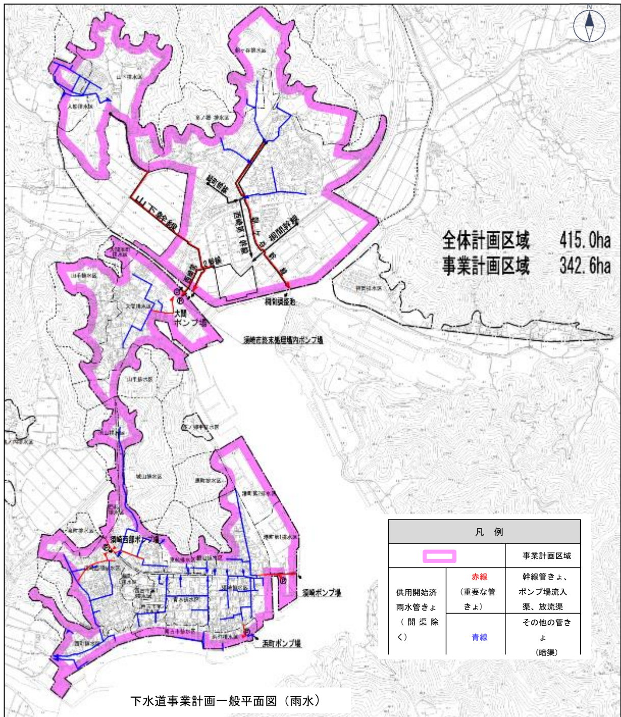
図 5-9 重要路線位置図
