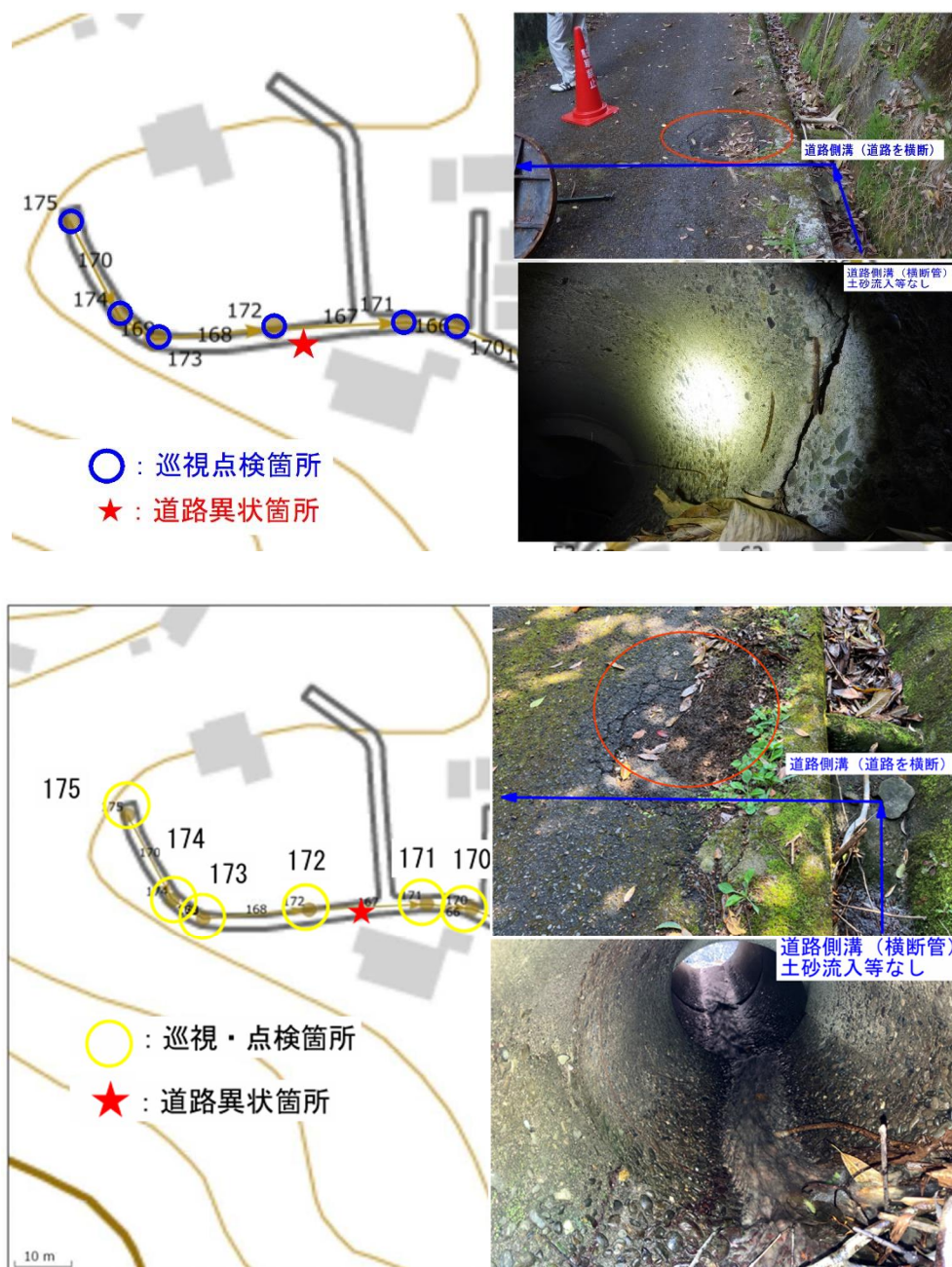
図 5-8 道路異状対象箇所図及び状況写真 (上) 令和7年度 (下) 令和8年度
