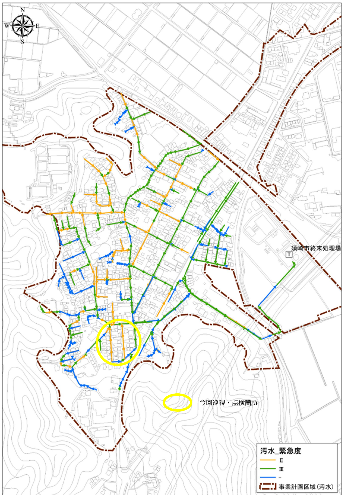
図 5-3 全体位置図
