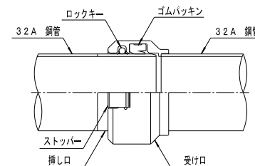
継手詳細図 S=FREE
