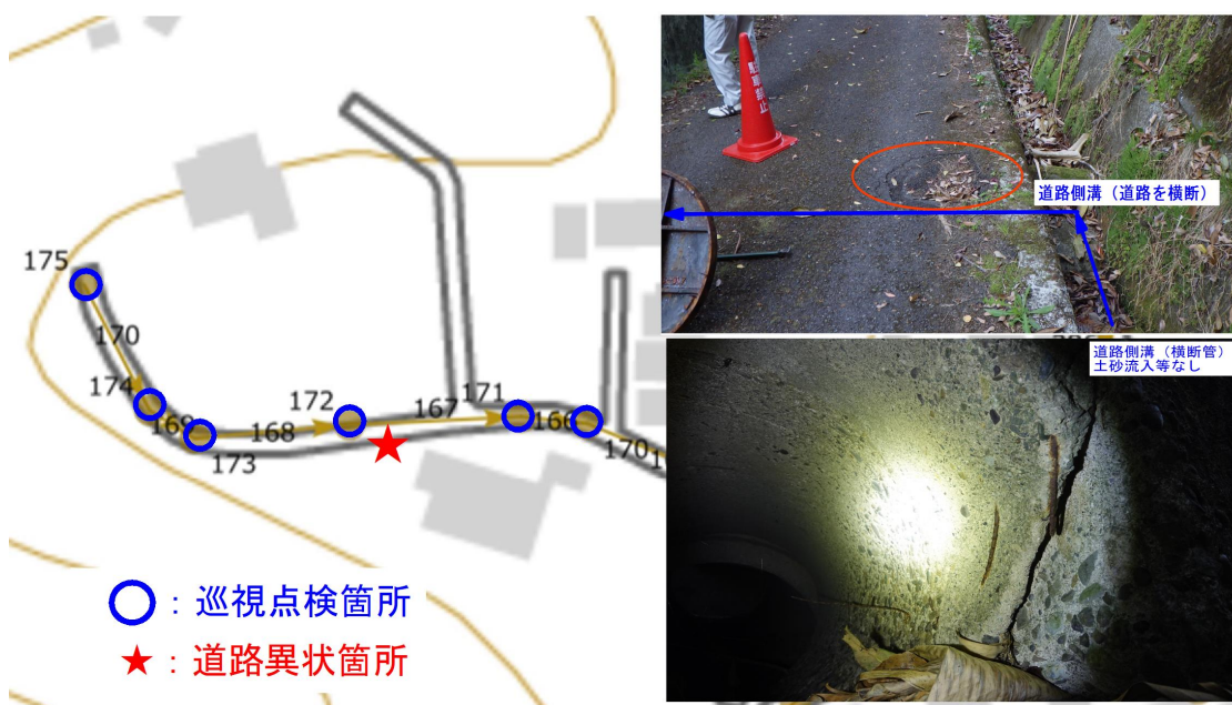
図 5.4 道路異状対象箇所図及び状況写真
