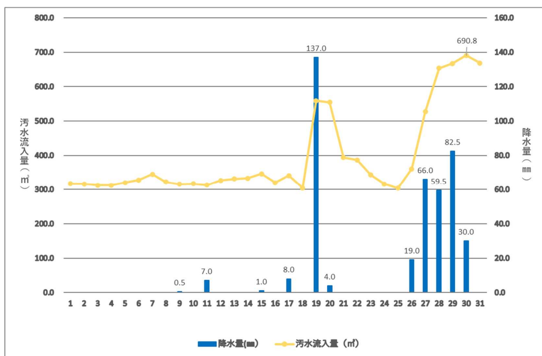
図 5.7 須崎市終末処理場の流入水量（令和6年8月）
