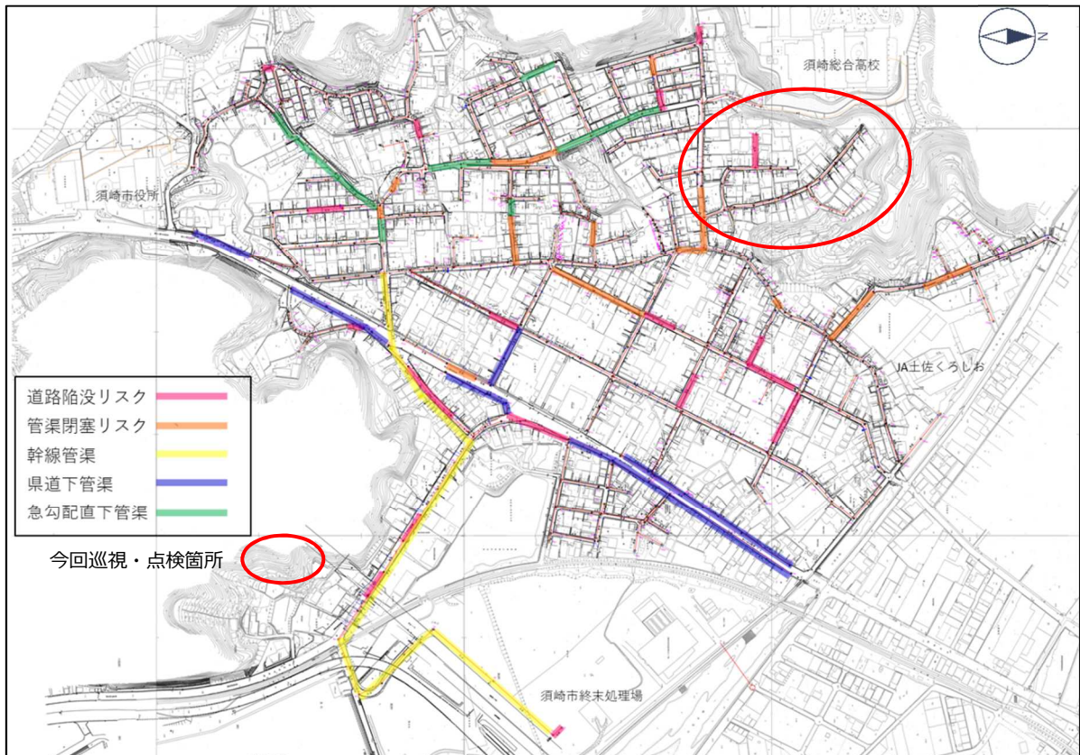
図 5.2 全体位置図
