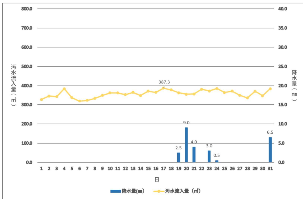
図 5.8 須崎市終末処理場の流入水量（R6 年 1 月）
