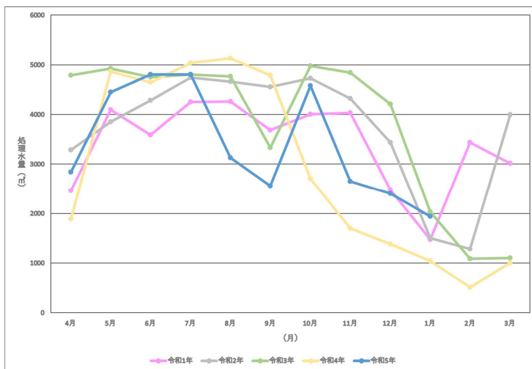
図 5.11 浸出水処理施設の処理水量の推移
