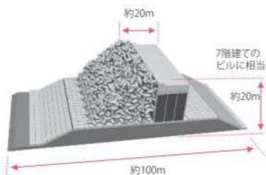
湾口地区津波防波堤のイメージ図
